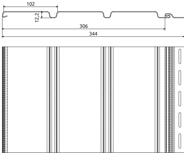
Панель суцільна (гладка)
