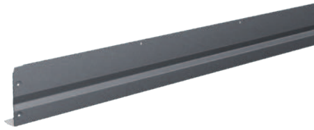
Планка вітрозахисту нижня WD 150 Л/П, WD 180 Л/П
