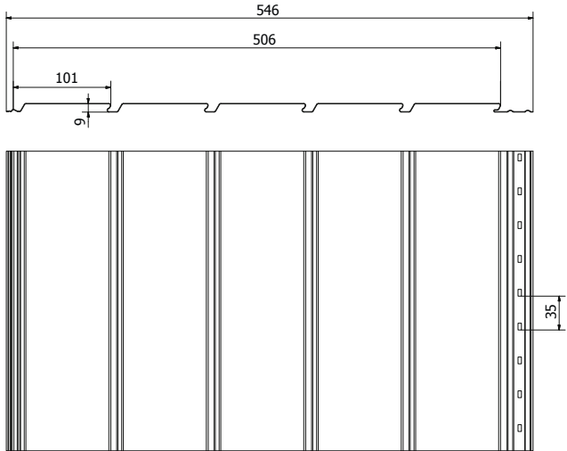
Панель суцільна (гладка)
