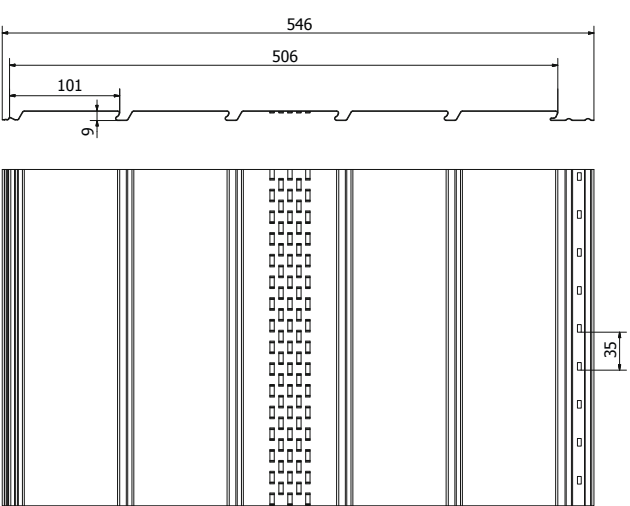
Панель вентильована (перфорована)
