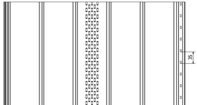
Панель вентилярована (перфорована)
