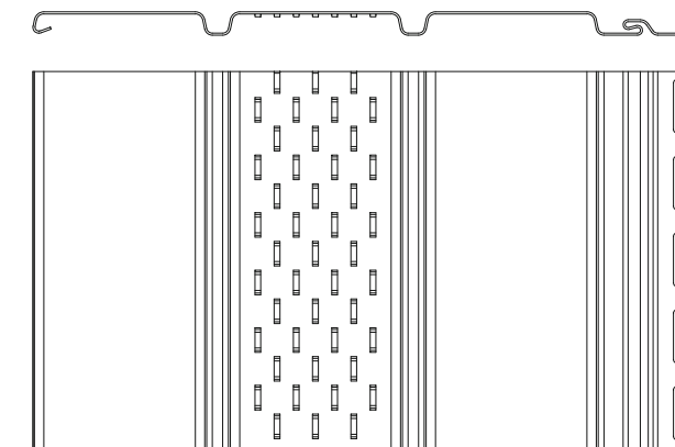
Панель вентильована (перфорована)
