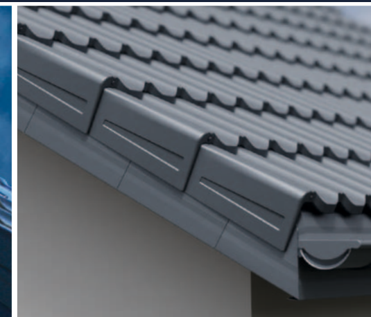
Модульна вітрова планка Venecja Drift - універсальна нижня вітрова планка
