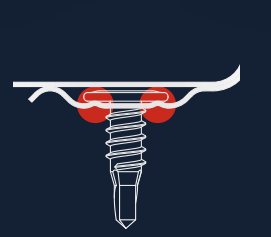
Спеціальні поздовжні хвиляподібні ребра жорсткості під капелюшок саморіза
