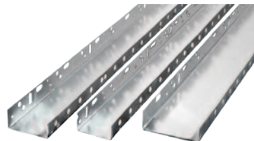
Профіль цокольний (стартовий) 2,5м WB 53, WB 63, WB 83, WB 103, WB 123, WB 153, WB 203
