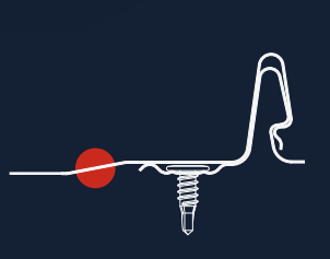
Піднята поверхня панелі, що утворює додаткове ребро жорсткості
