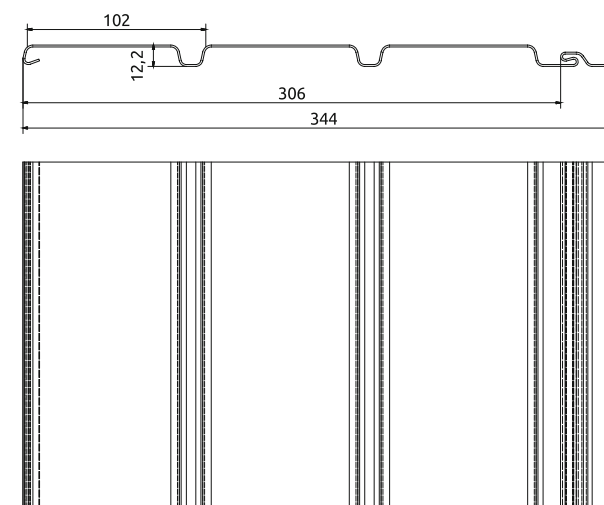
Панель суцільна (гладка)
